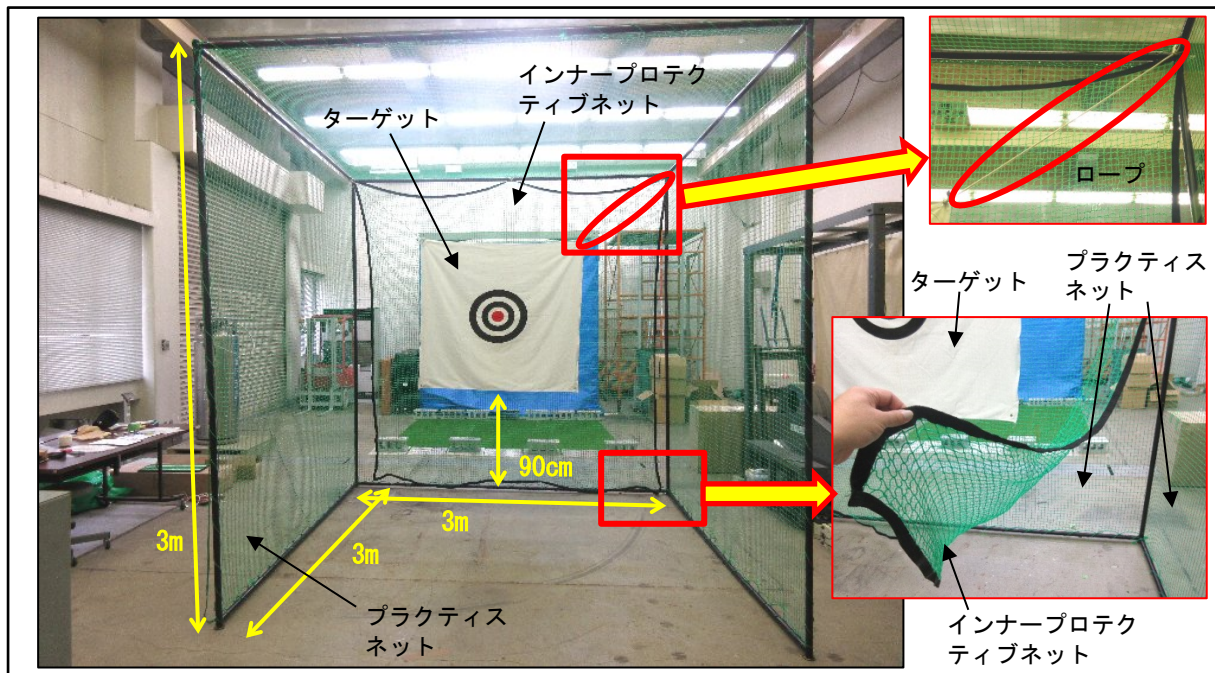
写真1. 当該品の外観（正面より観察）
