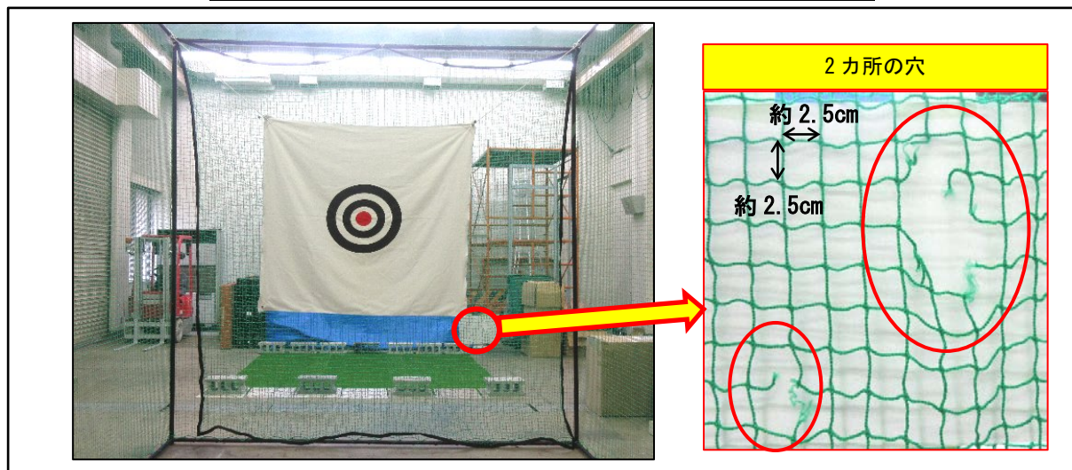
写真 2. インナープロテクティブネットの 2 カ所の穴の外観
