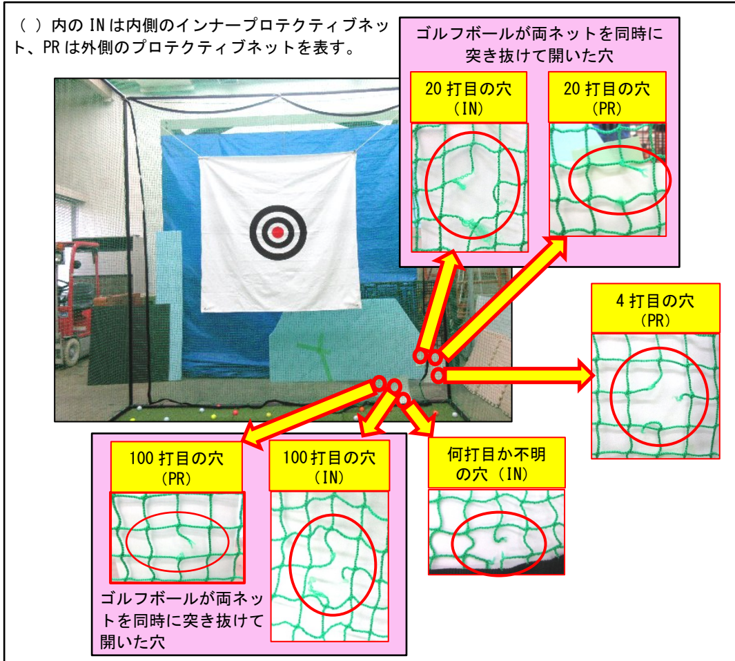
写真6. 実使用テストでモニターがゴルフボール100球を打ったときに開いた穴の外観
